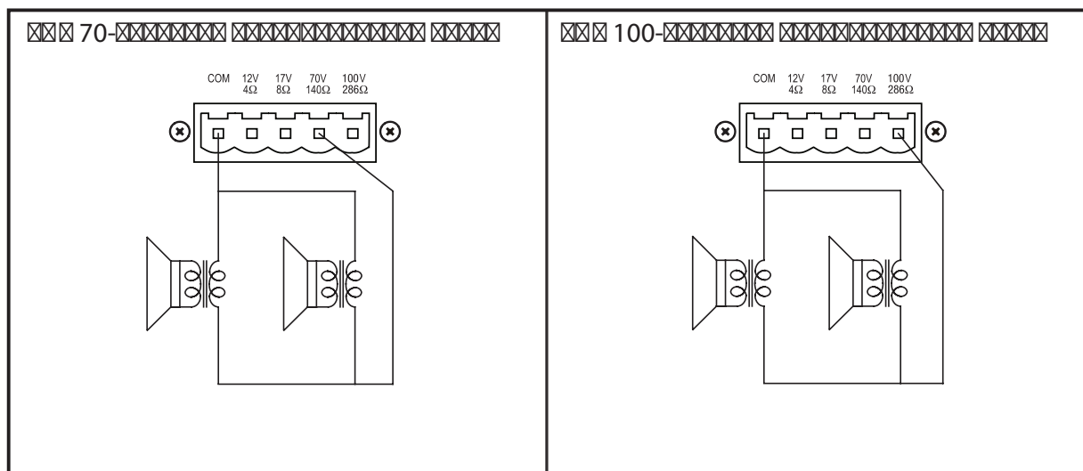
Схема подключения трансляционных линий 70 и 100 В.
